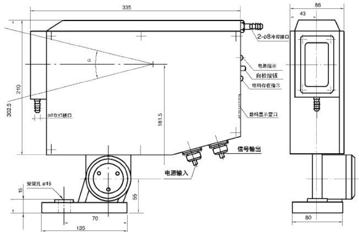
A 型活套检测器外形及安装尺寸
